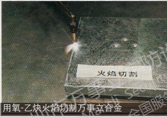
用氧-乙炔火焰切割万事立合金
